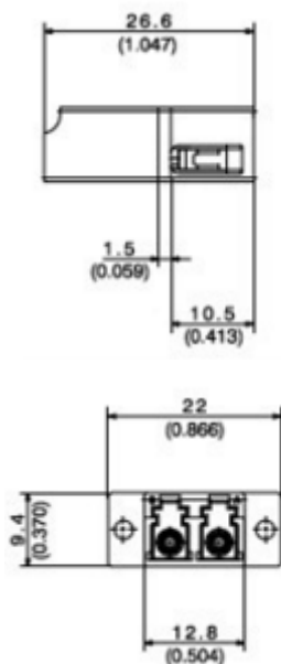
Adapter standardu LC duplex - wymiary
