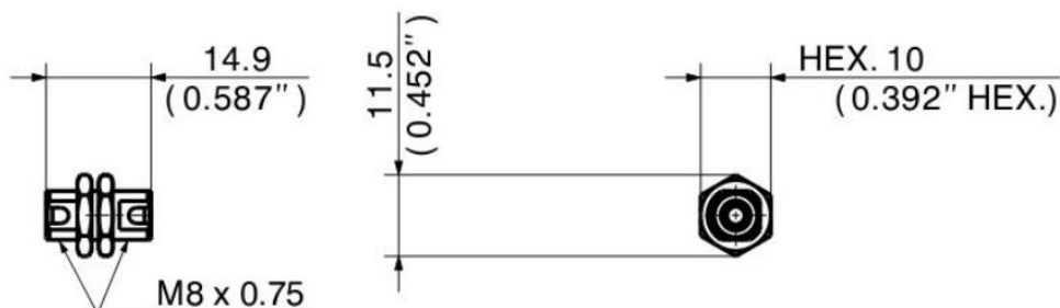
Zdjęcie i rysunek techniczny adaptera FC/PC SM (D-Shape)
