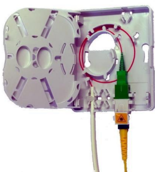
Gniazdo abonenckie serii CTB2-A
