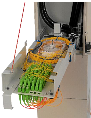
Szafka kablowa serii SUS-PH
